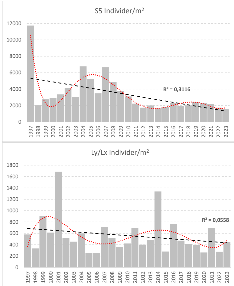
Figur 4. Individitæthet på station S5 i Skälderviken (överst) och station Ly i södra Laholmsbukten (underst) 1997-2023. Svart streckad linje anger linjär regression, röd punktlinje anger regression som polynom.
