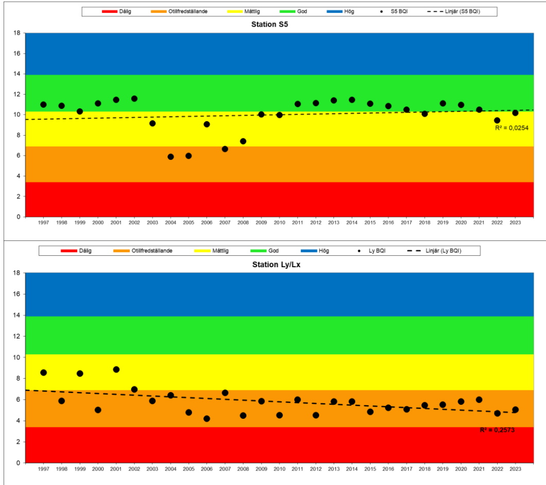
Figur 6. Benthic Quality Index (BQI) för station S5 i Skälderviken (överst) och station Ly/Lx i södra Laholmsbukten (underst) 1997-2023. 20-percentil för fem prov. Olika kvalitetsgränser för 5-20 meters djup inlagda. Linjär regression inlagd som streckad linje.
