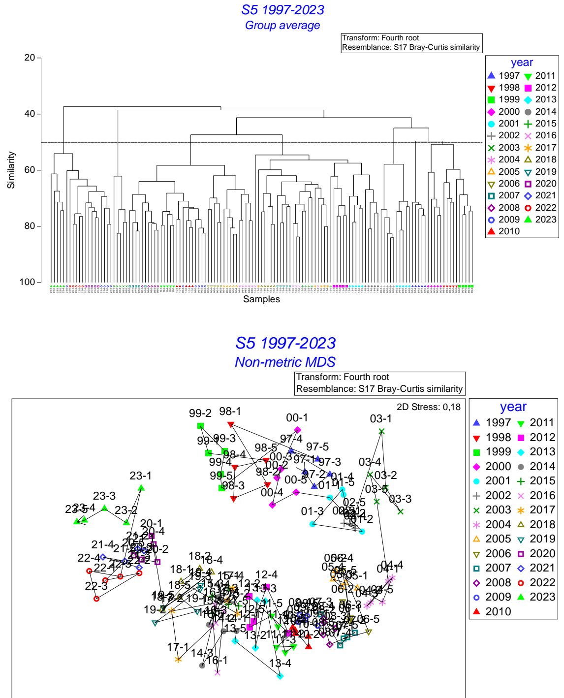
Figur 7. Utvecklingen på station S5 under perioden 1997-2023. Överst klusteranalys och underst MDS baserad på Bray-Curtis likhetskoefficient (dubbelrot-transformerade data).
