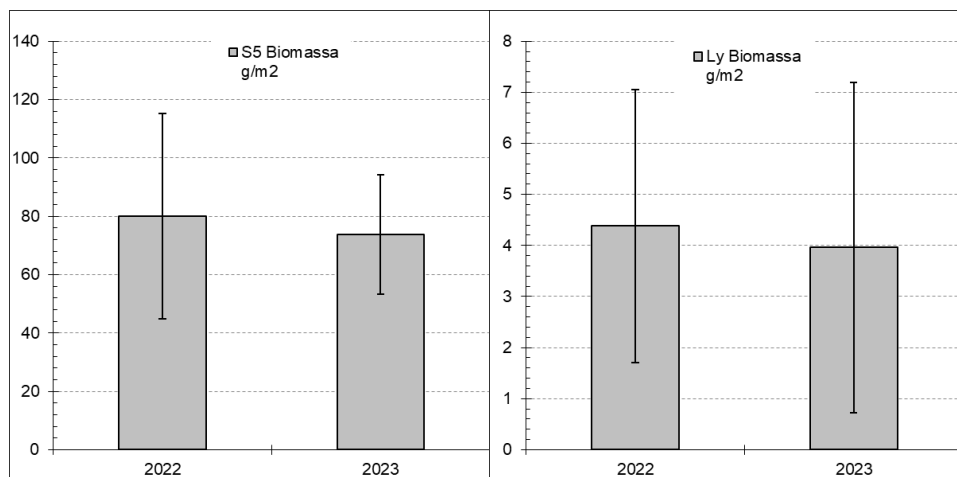
Figur 9. Biomassa (g/m 2 ) exklusive Arctica islandica för station S5 i Skälderviken (till vänster) och station Ly i södra Laholmsbukten (till höger) som undersökts 2022 och 2023. Staplar anger standardavvikelser.
