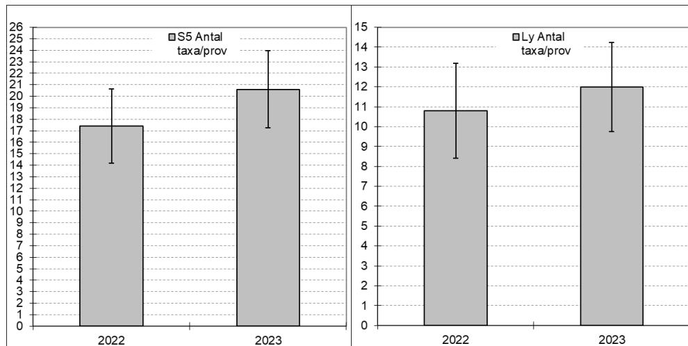
Figur 7. Antal taxa per prov för station S5 i Skälderviken (till vänster) och station Ly i södra Laholmsbukten (till höger) som undersökts 2022 och 2023. Staplar anger standardavvikelser.
