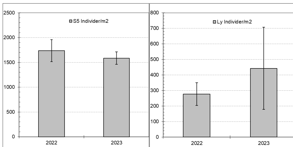
Figur 8. Individdtäthet (ind/m 2 ) för station S5 i Skälderviken (till vänster) och station Ly i södra Laholmsbukten (till höger) som undersökts 2022 och 2023. Staplar anger standardavvikelser.
