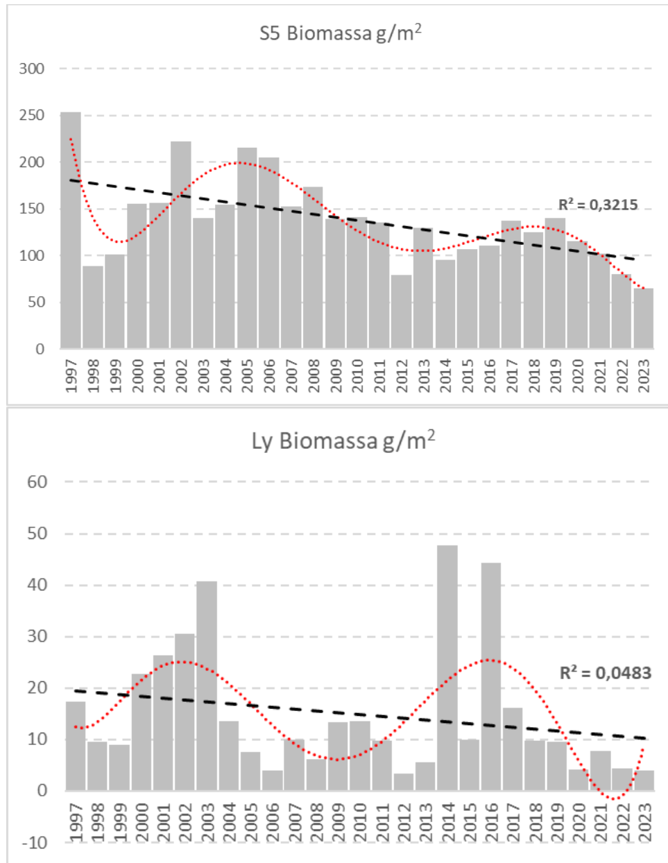
Figur 5. Biomassan på station S5 i Skälderviken (överst) och station Ly i södra Laholmsbukten (underst) 1997-2023. Svart streckad linje anger linjär regression, röd punktlinje anger regression som polynom.
