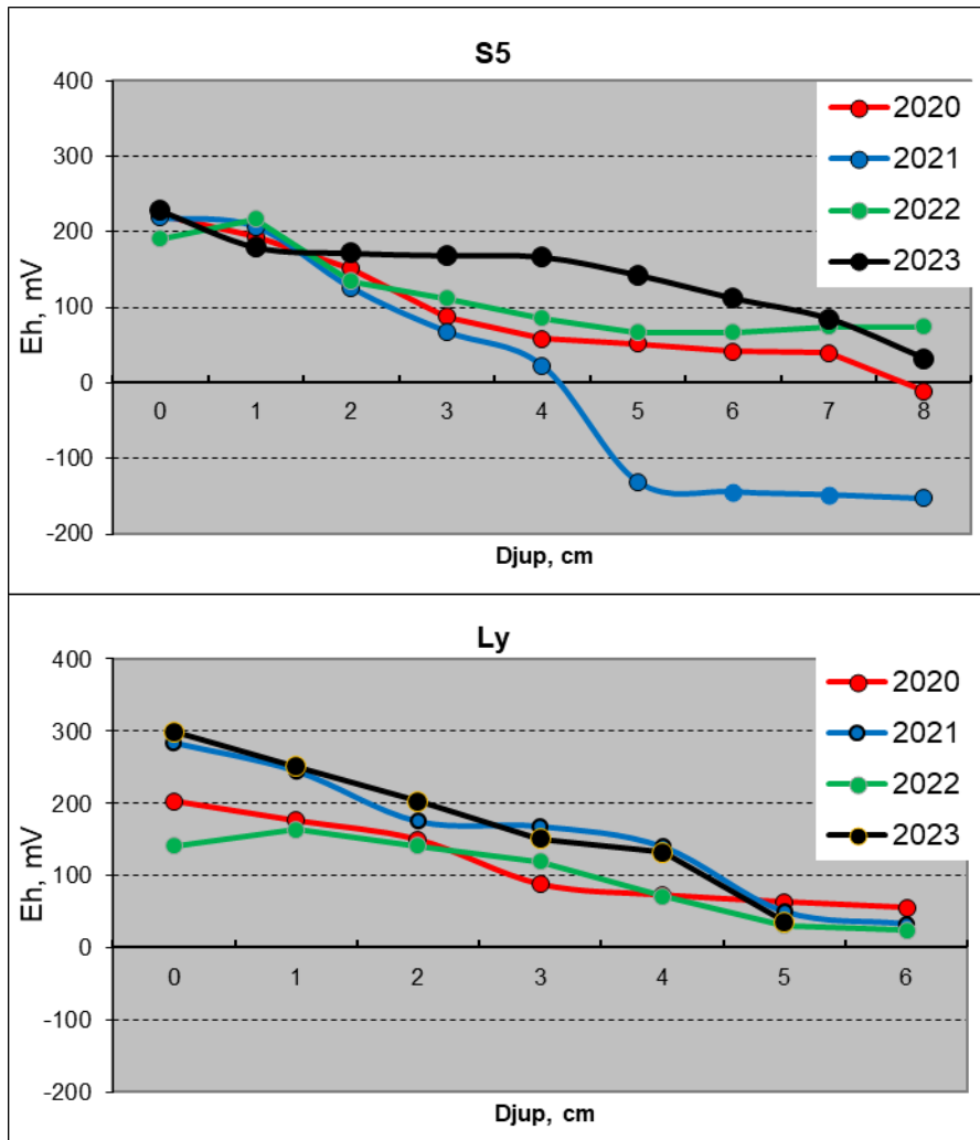
Figur 2. Redoxpotential (Eh, mV) på olika djup i sedimentet på stationerna S5 och Ly 2020- 2023.
