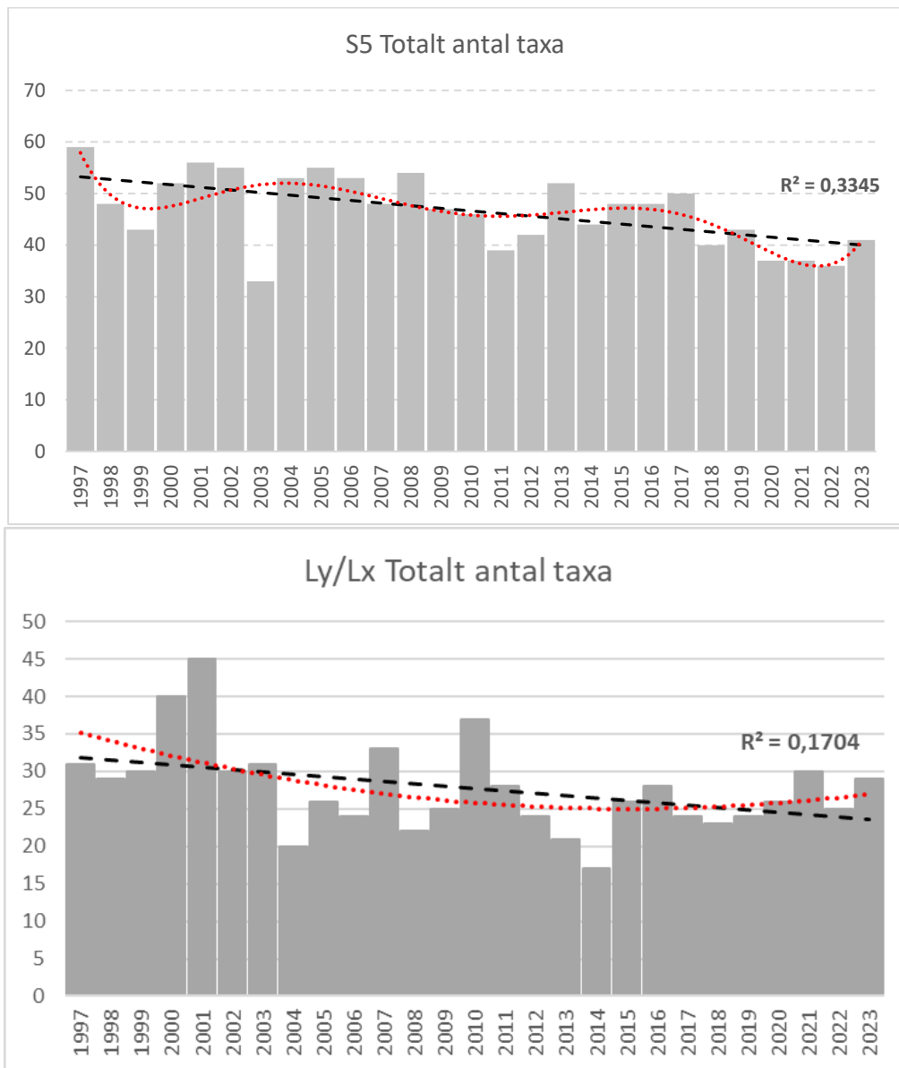
Figur 3. Totalt antal taxa på station S5 i Skälderviken (överst) och station Ly i södra Laholmsbukten (underst) 1997-2023. Svart streckad linje anger linjär utveckling, röd punktlinje anger utveckling som polynom.
