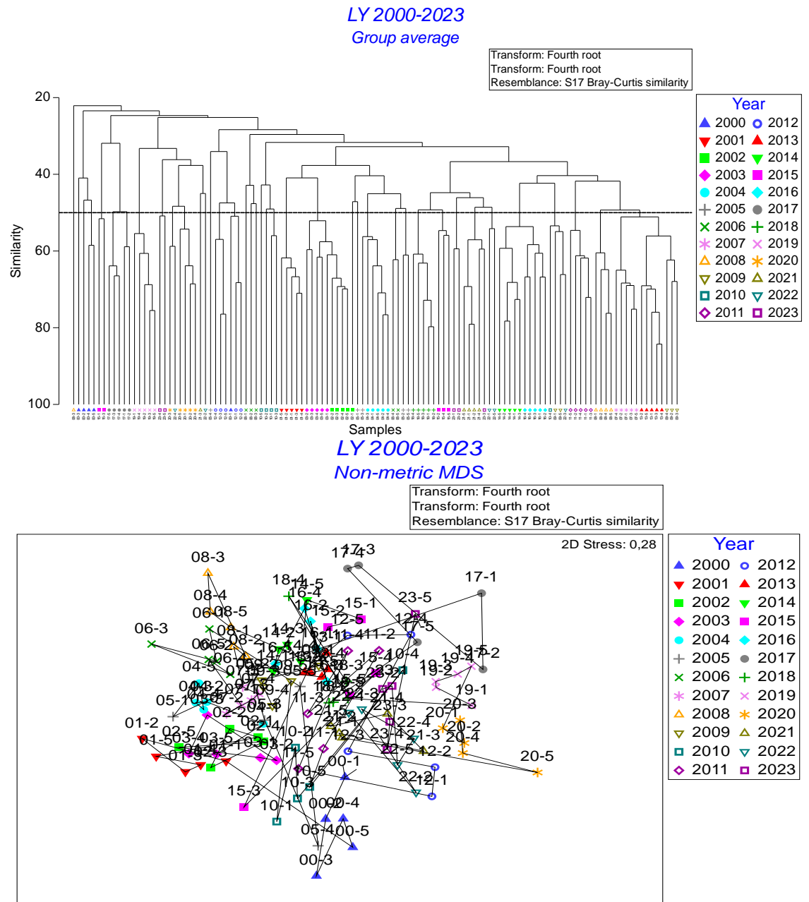
Figur 8. Utvecklingen på station Ly under perioden 2000-2023. Överst klusteranalys och underst MDS baserad på Bray-Curtis likhetskoefficient (dubbelrot-transformerade data).
