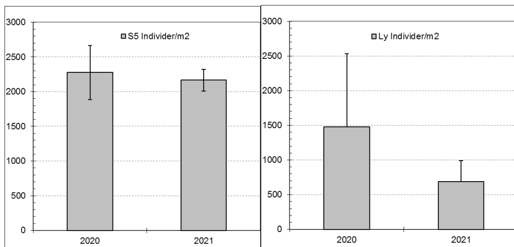
Figur 8. Individtäthet (ind/m 2 ) för station S5 i Skälderviken (till vänster) och station Ly i södra Laholmsbukten (till höger) som undersökts 2020 och 2021. Staplar anger standardavvikelser.
