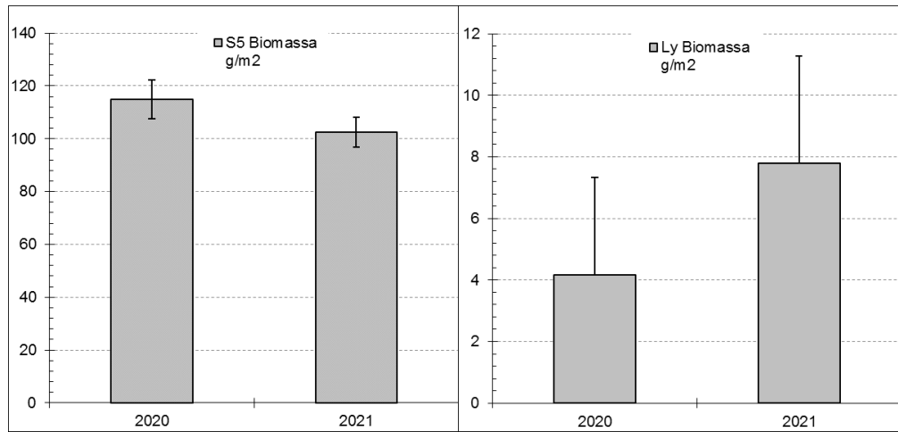
Figur 9. Biomassa (g/m 2 ) exklusive Arctica islandica för station S5 i Skälderviken (till vänster) och station Ly i södra Laholmsbukten (till höger) som undersökts 2020 och 2021. Staplar anger standardavvikelser.
