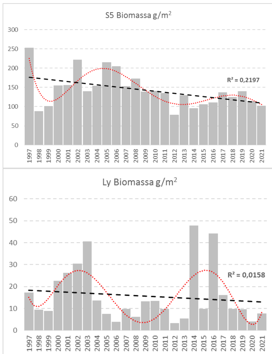
Figur 5. Biomassan på station S5 i Skälderviken 1997-2021 (överst) och station Ly i södra Laholmsbukten (underst). Svart streckad linje anger linjär regression, röd punktlinje anger regression som 6:e ordningens polynom.
