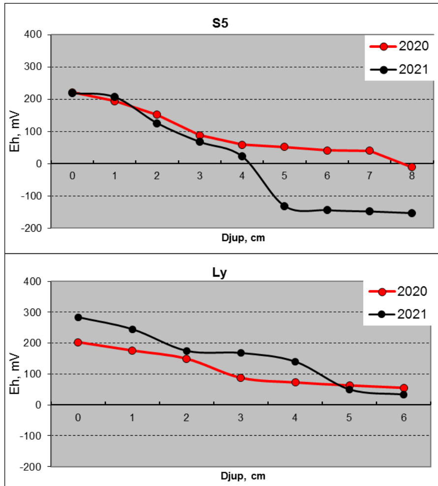
Figur 2. Redoxpotential (Eh, mV) på olika djup i sedimentet på stationerna S5 och Ly 2020 och 2021.
