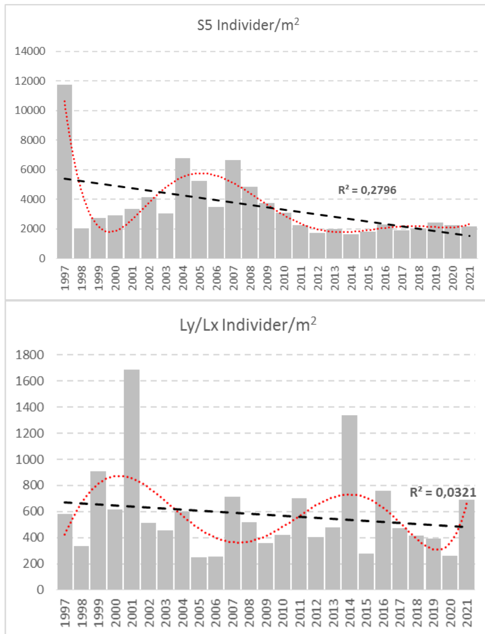
Figur 4. Individtäthet på station S5 i Skälderviken 1997-2021 (överst) och station Ly i södra Laholmsbukten (underst). Svart streckad linje anger linjär regression, röd punktlinje anger regression som 6:e ordningens polynom.
