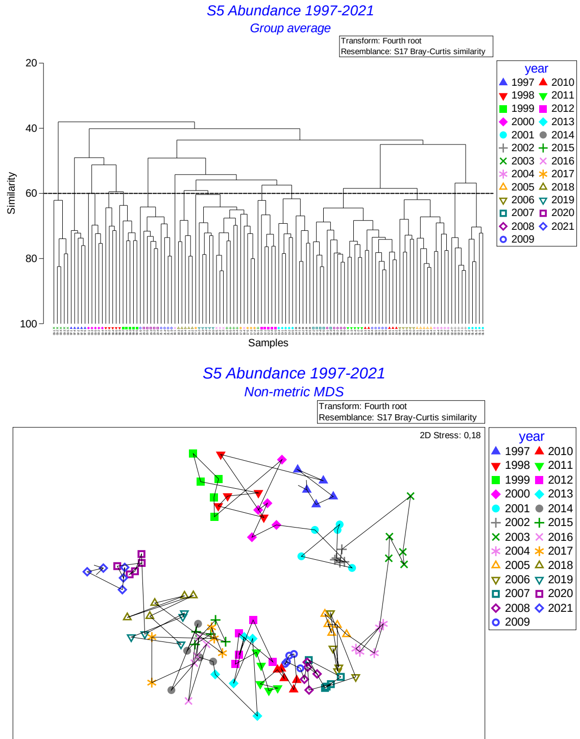
Figur 7. Utvecklingen på station S5 under perioden 1997-2021. Överst klusteranalys och underst MDS baserad på Bray-Curtis likhetskoefficient (dubbelrot-transformerade data).
