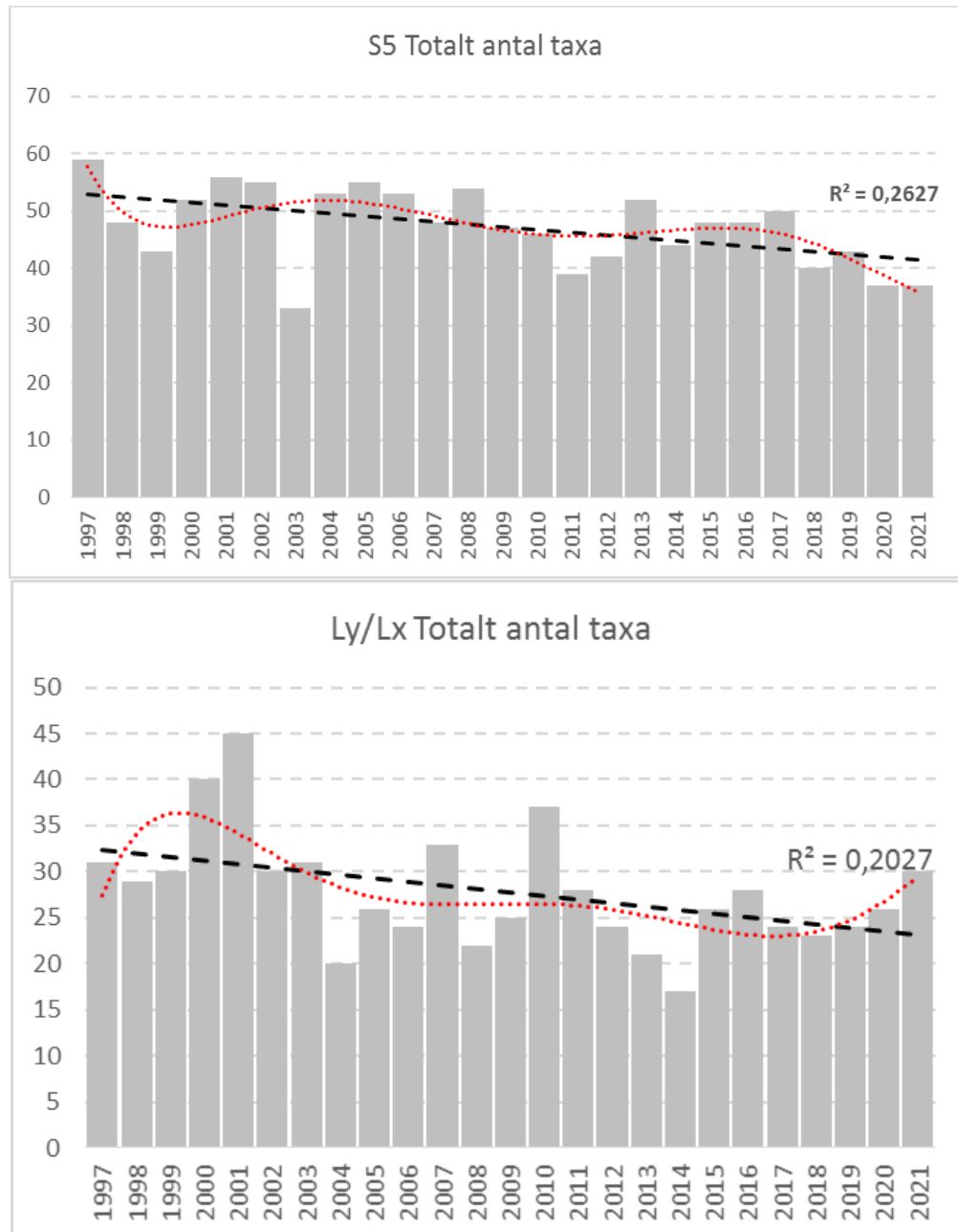
Figur 3. Totalt antal taxa på station S5 i Skälderviken 1997-2021 (överst) och station Ly i södra Laholmsbukten (underst). Svart streckad linje anger linjär regression, röd punktlinje anger regression som 6:e ordningens polynom.
