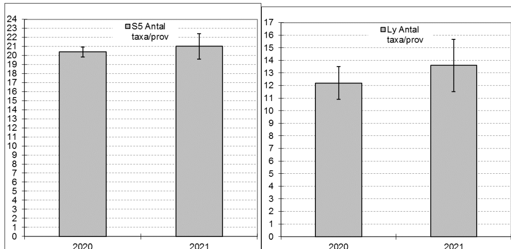
Figur 7. Antal taxa per prov för station S5 i Skälderviken (till vänster) och station Ly i södra Laholmsbukten (till höger) som undersökts 2020 och 2021. Staplar anger standardavvikelser.
